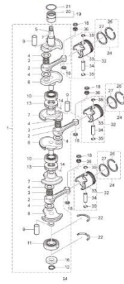
Fig. 2 Piston • Crank Shaft
