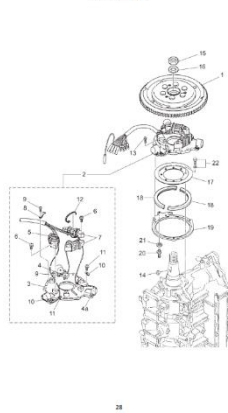
Fig. 8 Magneto
