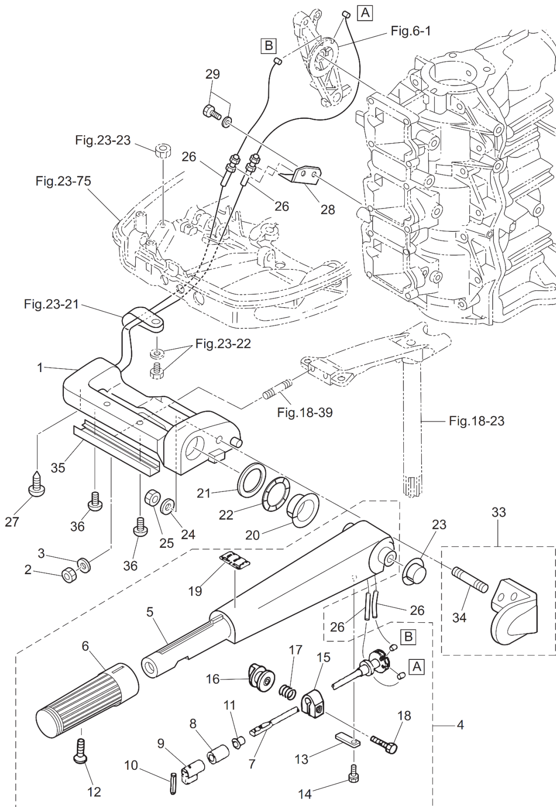
Fig. 22 Tiller Handle
