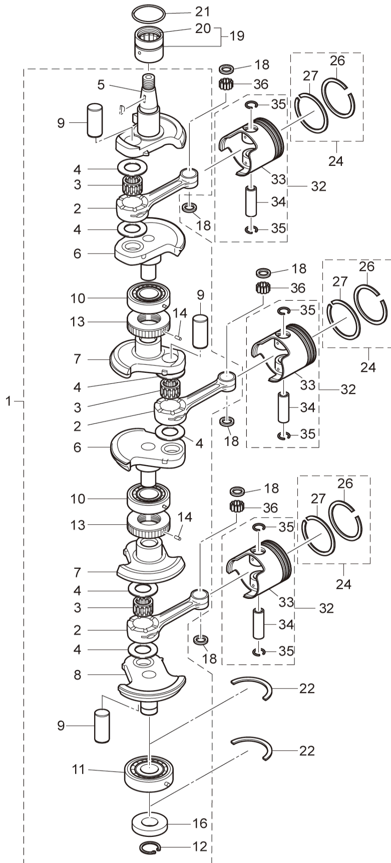
Fig. 2 Piston • Crank Shaft
