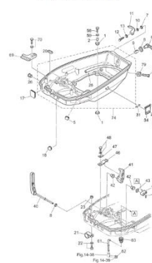
Fig. 23 Bottom Cowl • Shift
