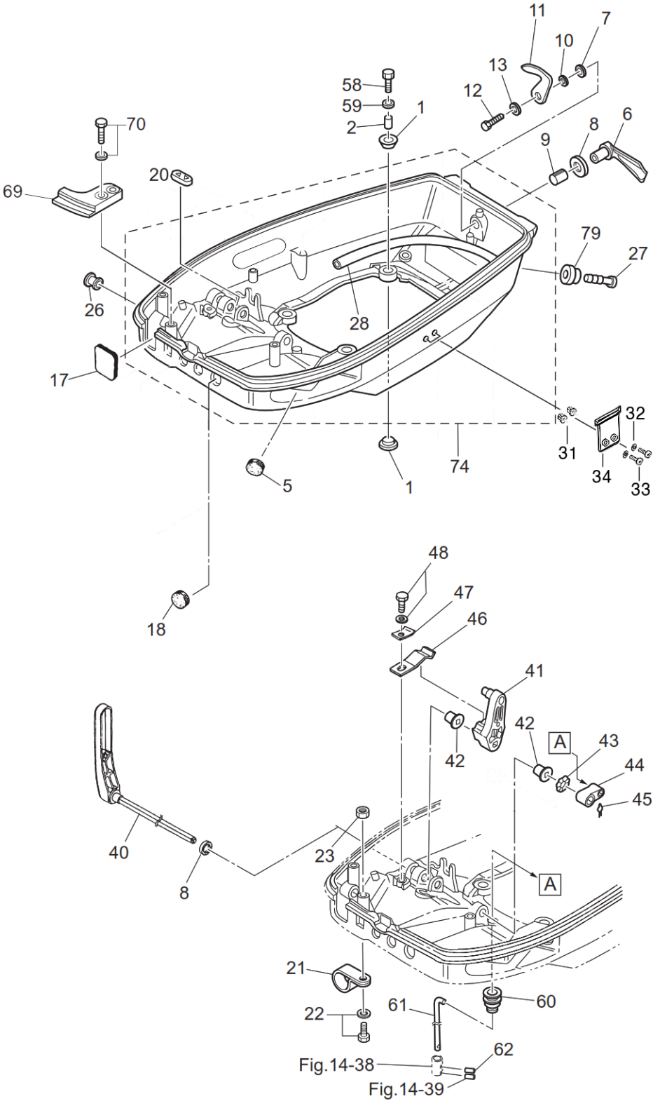
Fig. 23 Bottom Cowl • Shift
