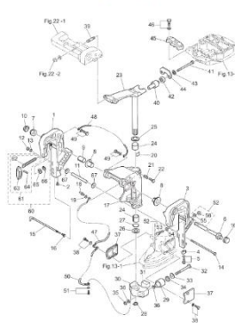
Fig. 18 Bracket (Manual Tilt)
