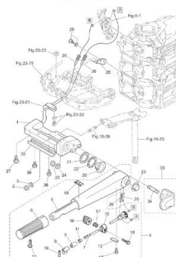
Fig. 22 Tiller Handle
