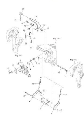
Fig. 19 Manual Tilt
